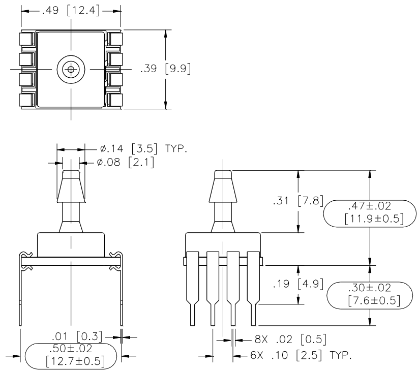
Model: MS4525DO-TPvoixxyP
